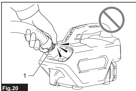
► 1. Raccord de tuyau
